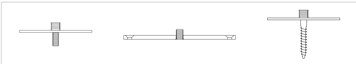
rocketbase concrete (Lastverteilplatte für Beton)
